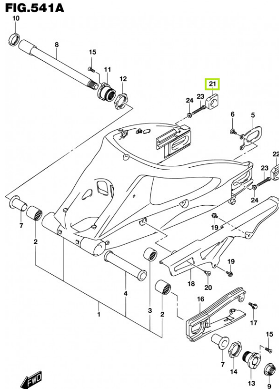
GSX-R1000L5_E21_541A REAR SWINGARM
