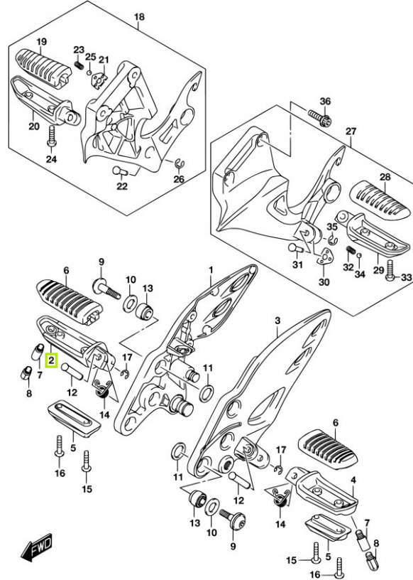
FIG.415A
